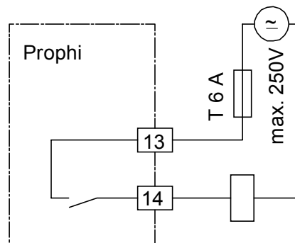
Zapojovací schéma alarmového výstupu
