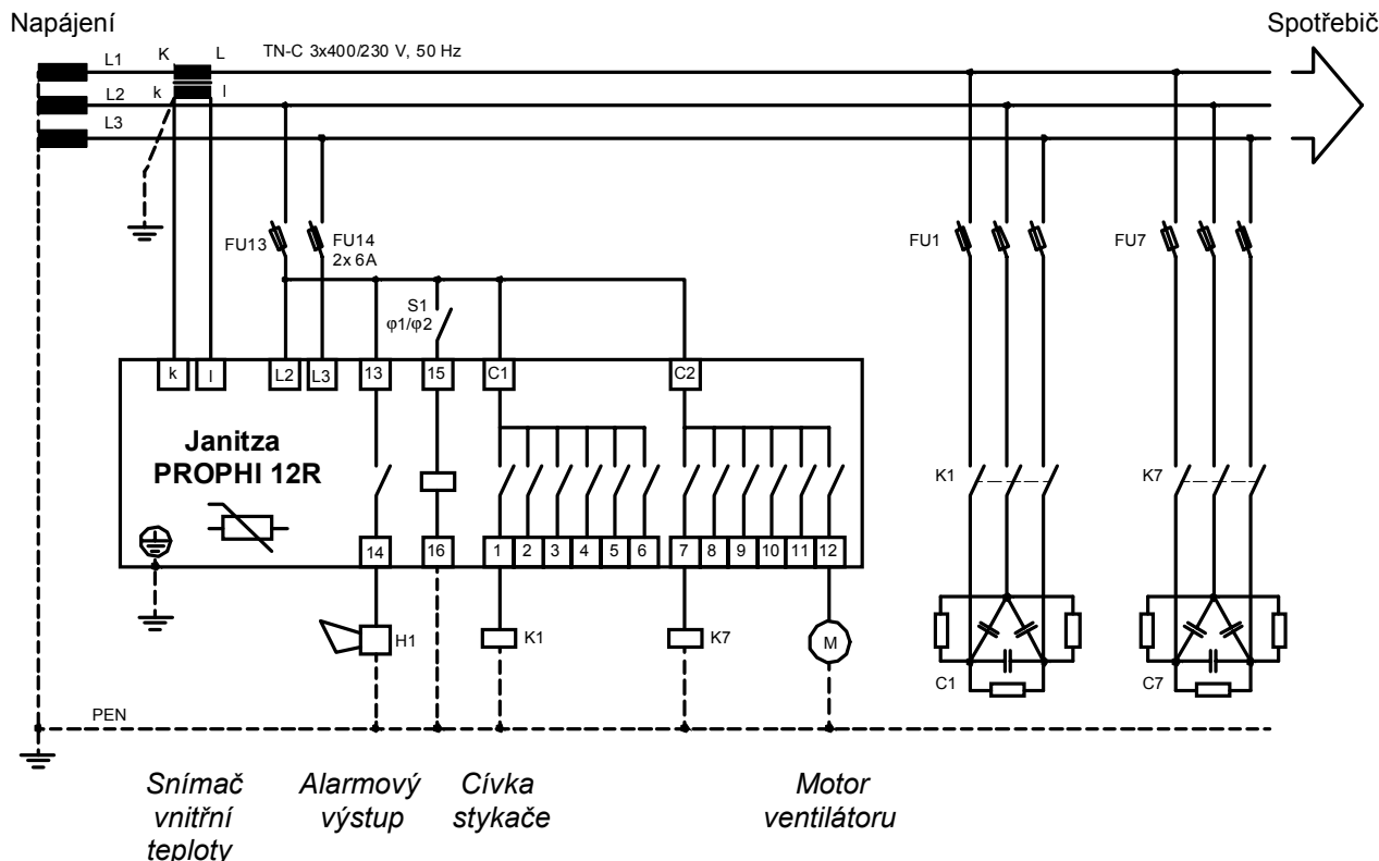
Příklad zapojení regulátoru jalového výkonu s připojeným motorem ventilátoru
