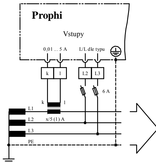
Připojení měřícího a pomocného napětí a transformátoru proudu
