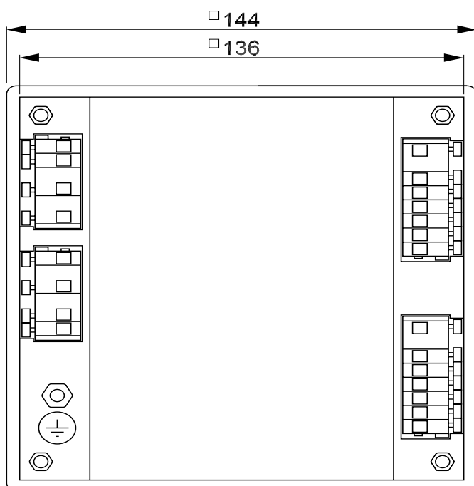
Pohled zezadu
